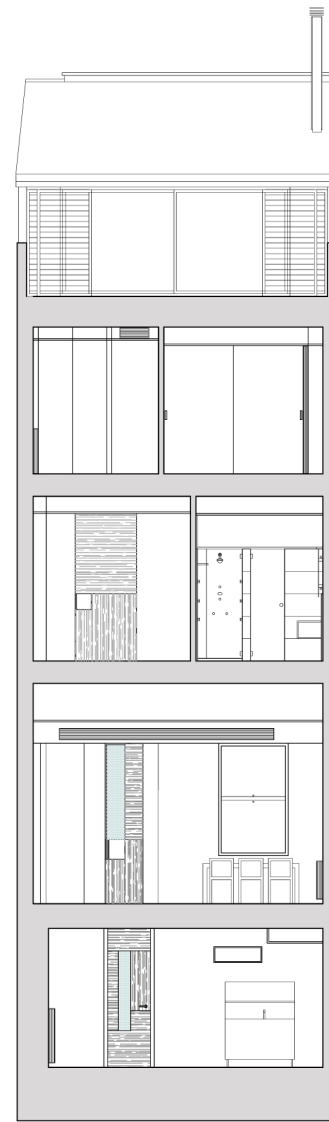
SECCIÓ E-E' SECCIÓ E-E'
