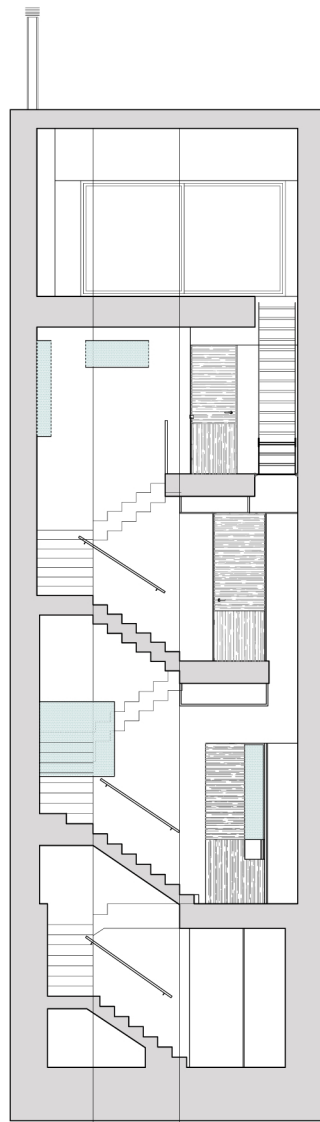
SECCIÓ D-D' SECCIÓ D-D'
