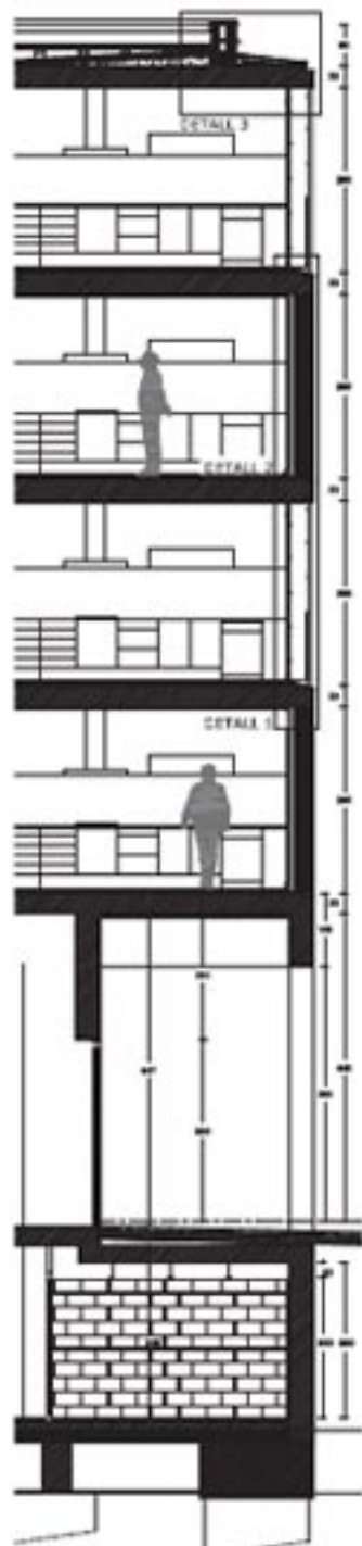
SECCIÓ CONSTRUCTIVA
