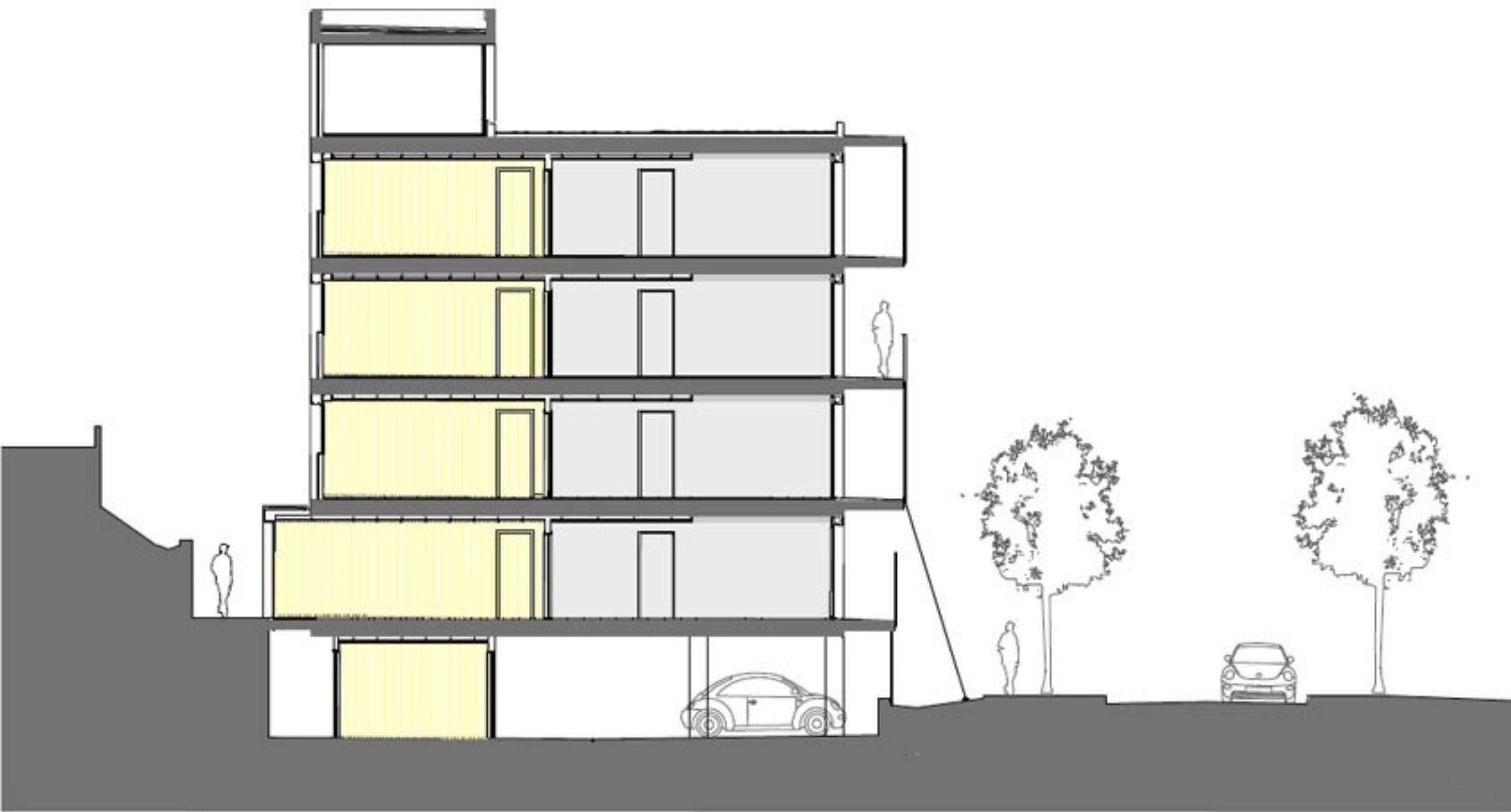
SECCIÓ TRANSVERSAL
