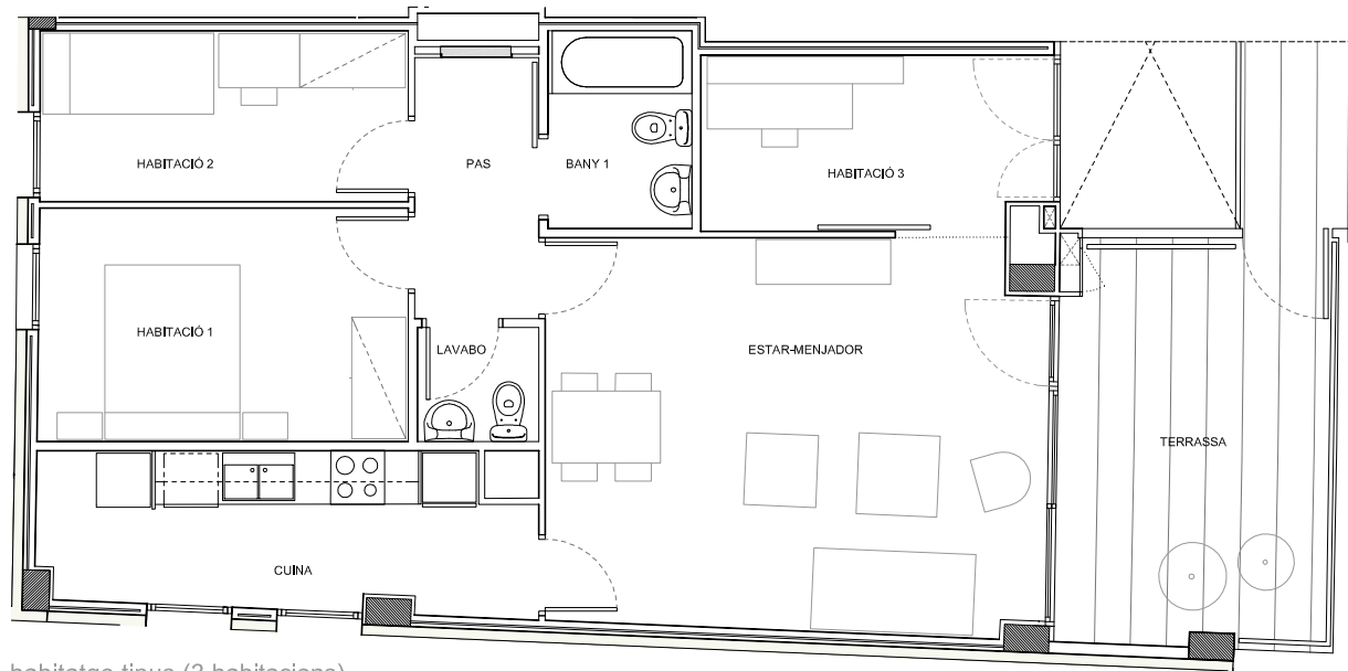
habitatge tipus (3 habitacions)
