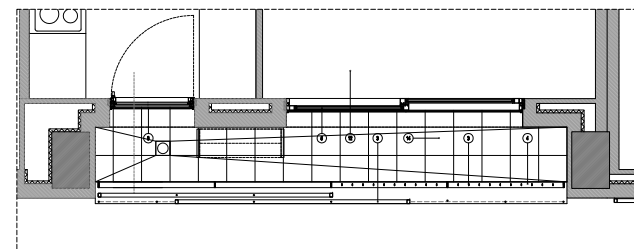
DETALLS CONSTRUCTIUS BALCONS
