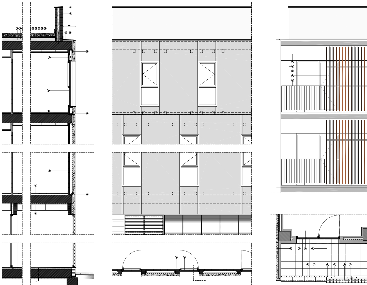
DETALLS CONSTRUCTIUS FAÇANA TESTER
