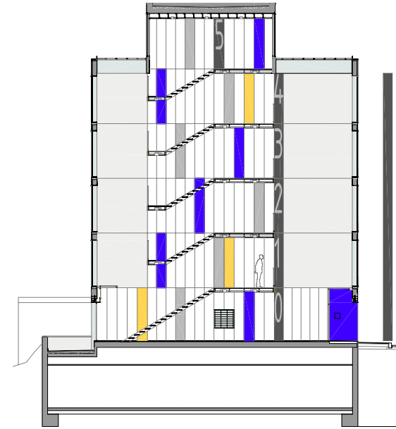
SECCIÓ V1
