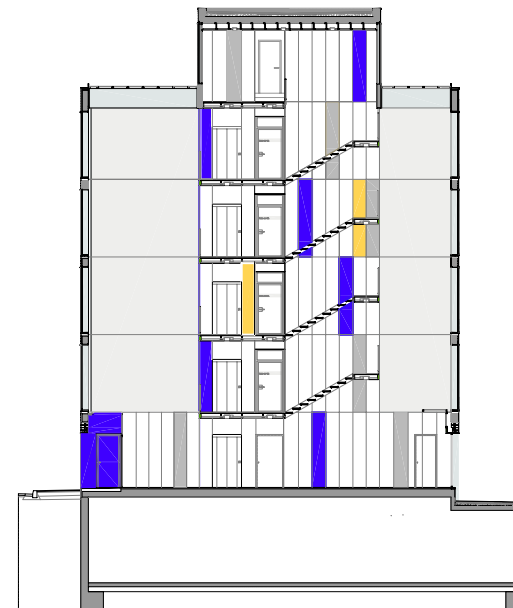
SECCIÓ V2
