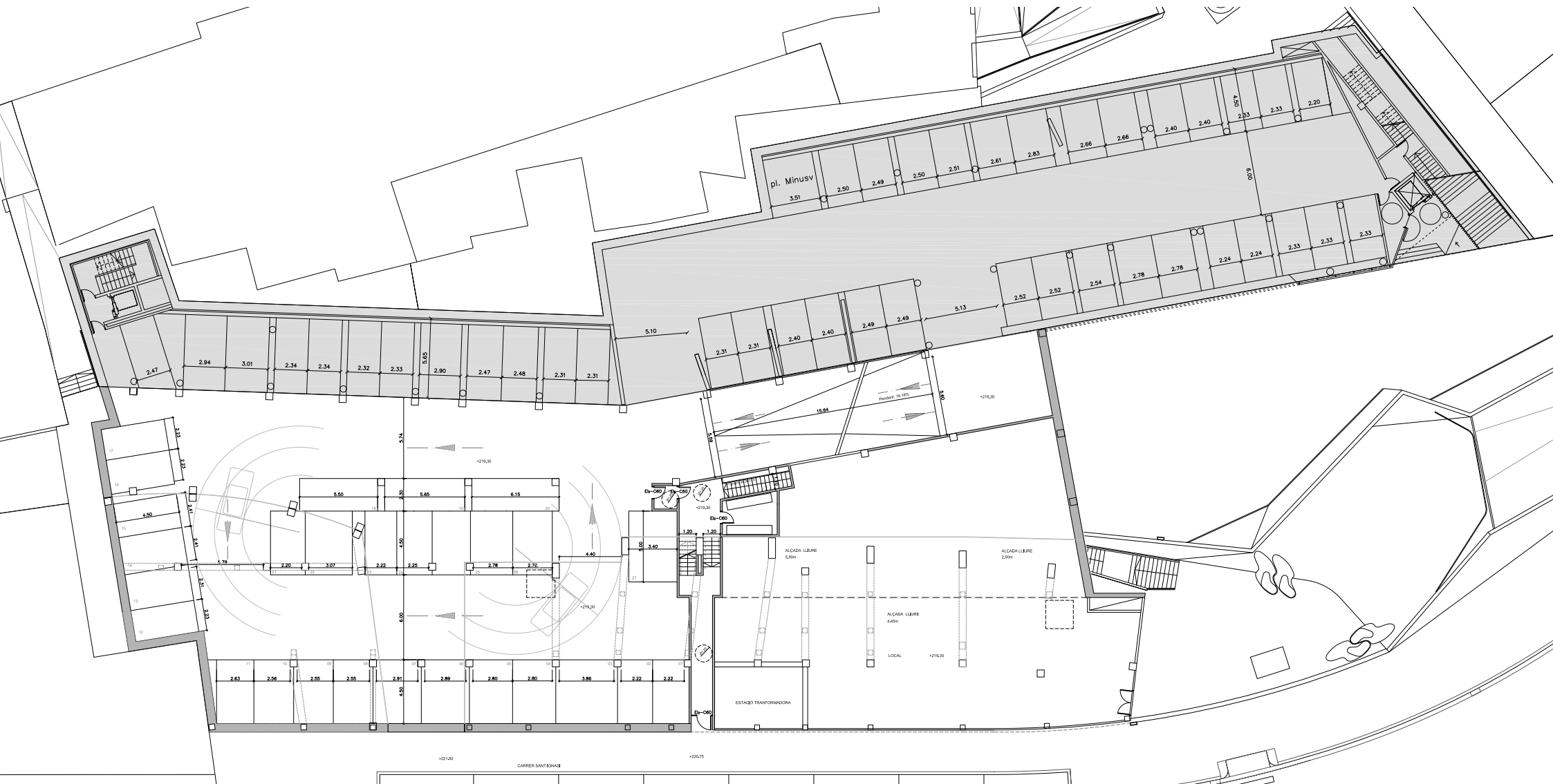
Planta Aparcament
