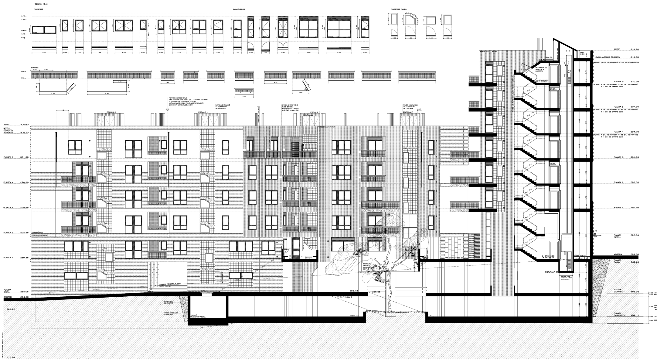
SECCIÓ D: LONGITUDINAL PER PATI I
