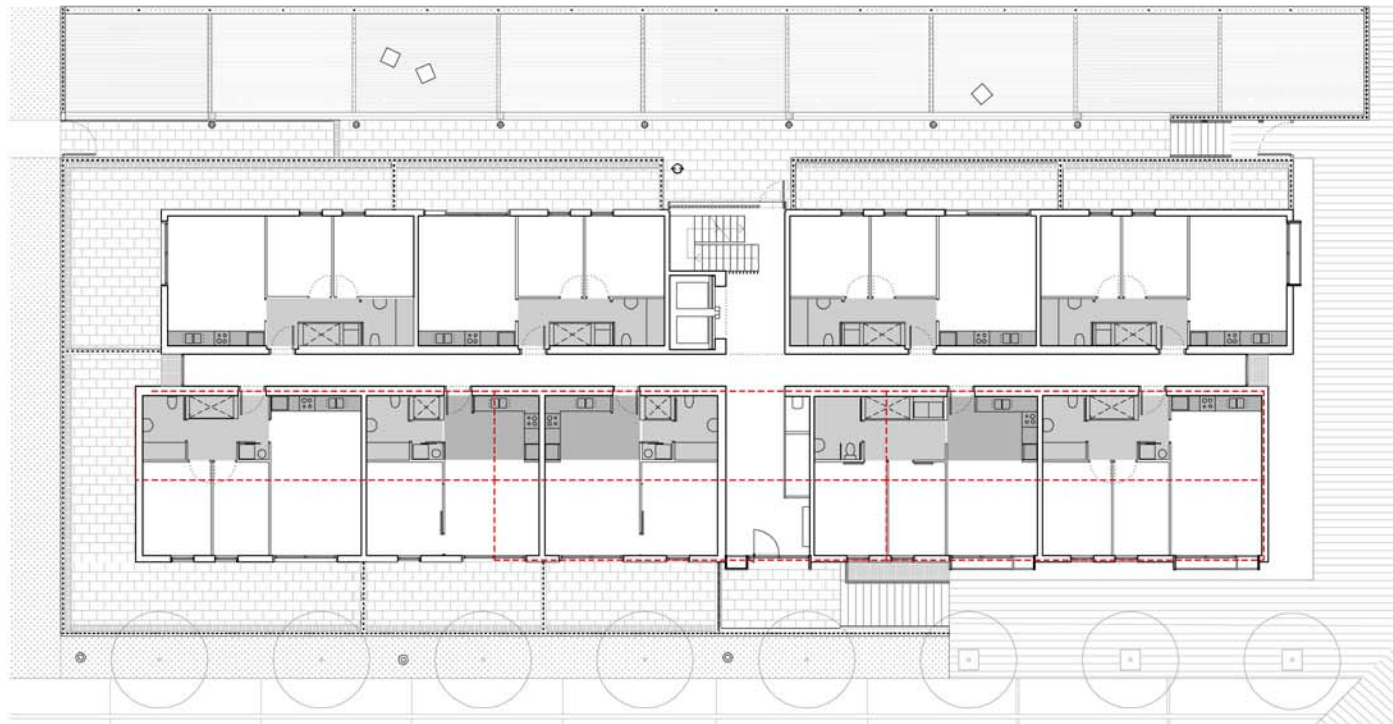
PB PLANTA BAIXA
