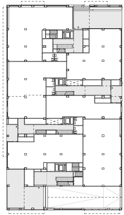
0 10 Planta baixa
