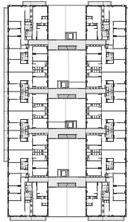
0 10 Planta tipus
