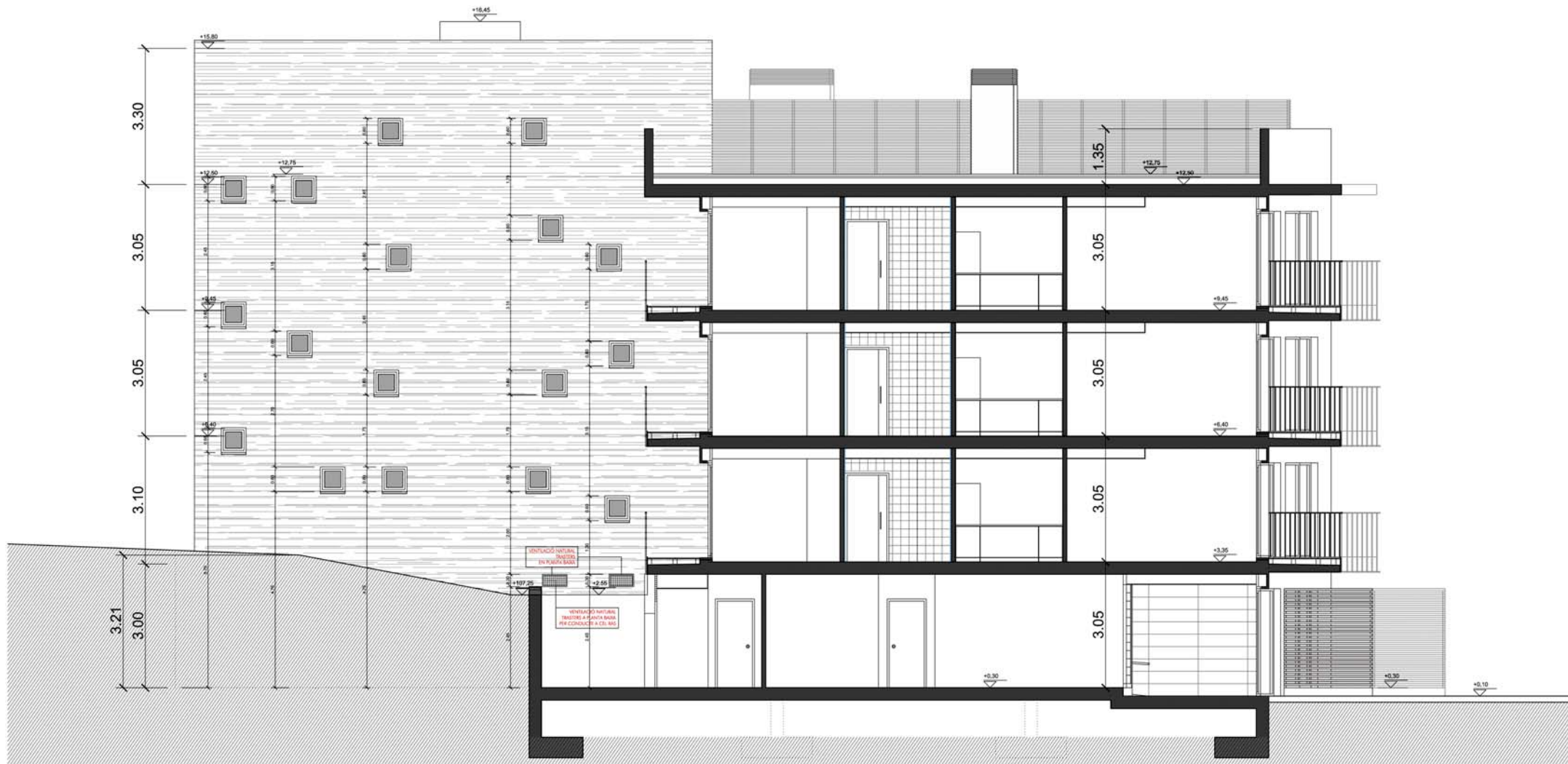
SECCIÓ D-D' EDIFICI D - PROMUNSA - SANT JUST
