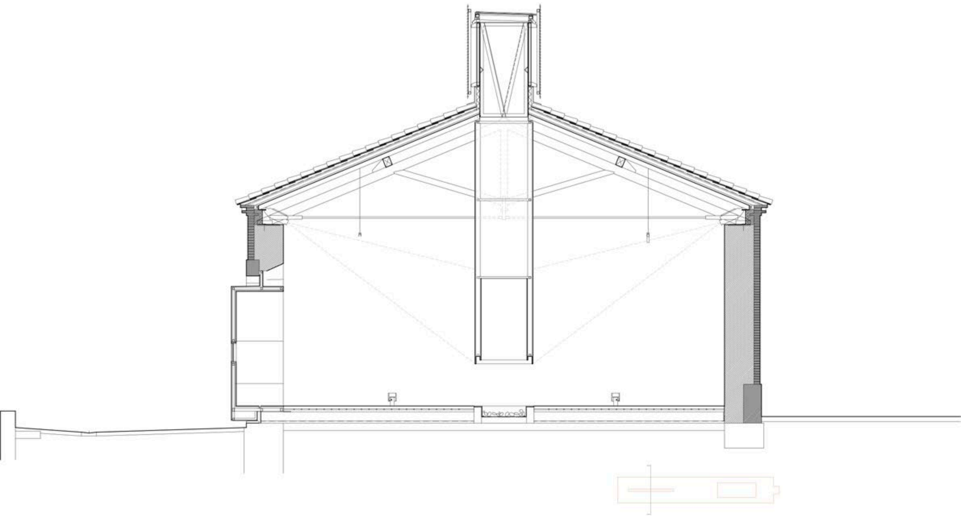
SECCIÓN POR EL ESPACIO DE EXPOSICIÓN PERMANENTE_
