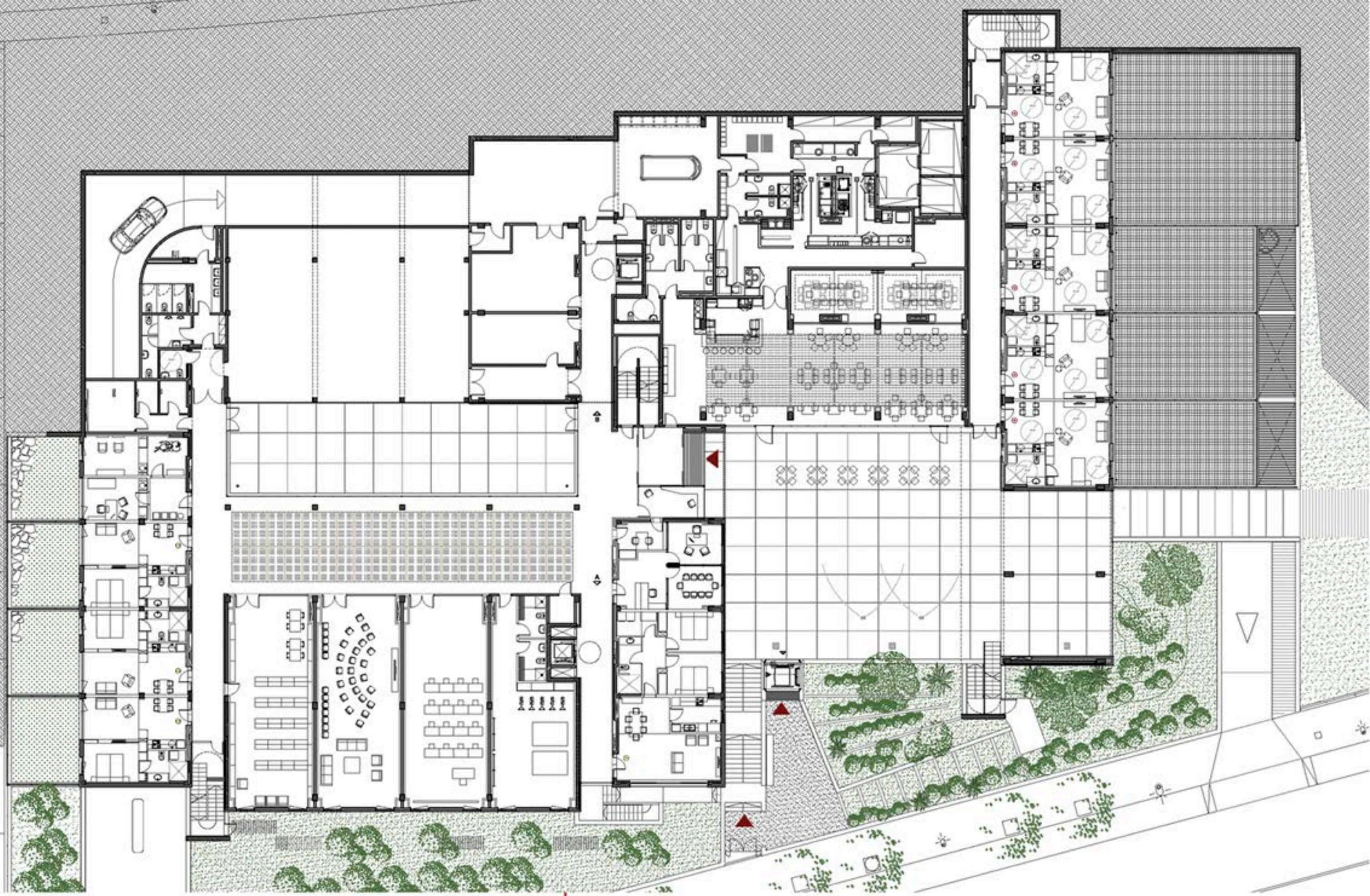
Planta baixa
