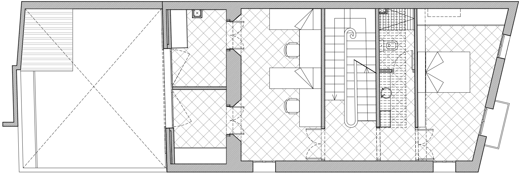
PLANTA PRIMERA
