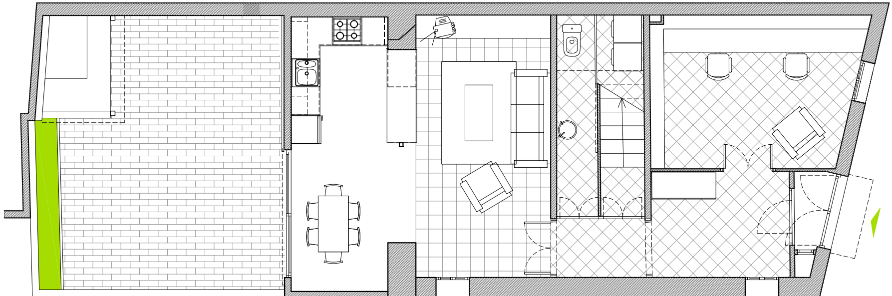
PLANTA BAIXA
