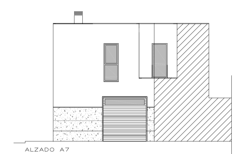
ALZADO A7
