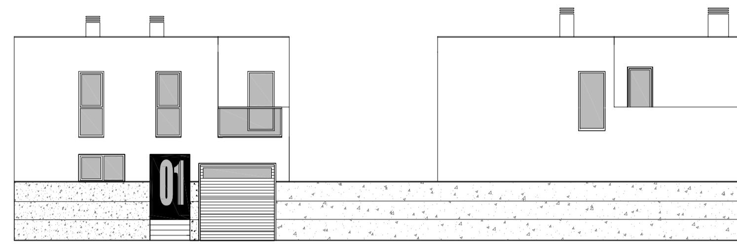
ALZADO A8
