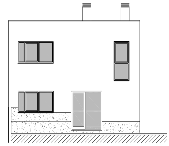
ALZADO A11
