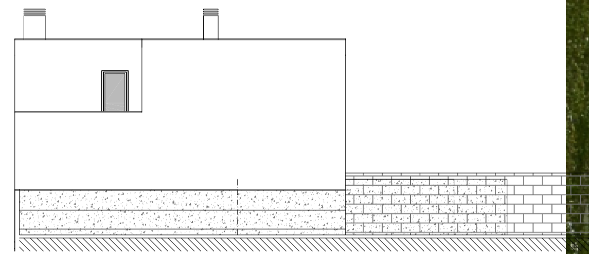
ALZADO A4
