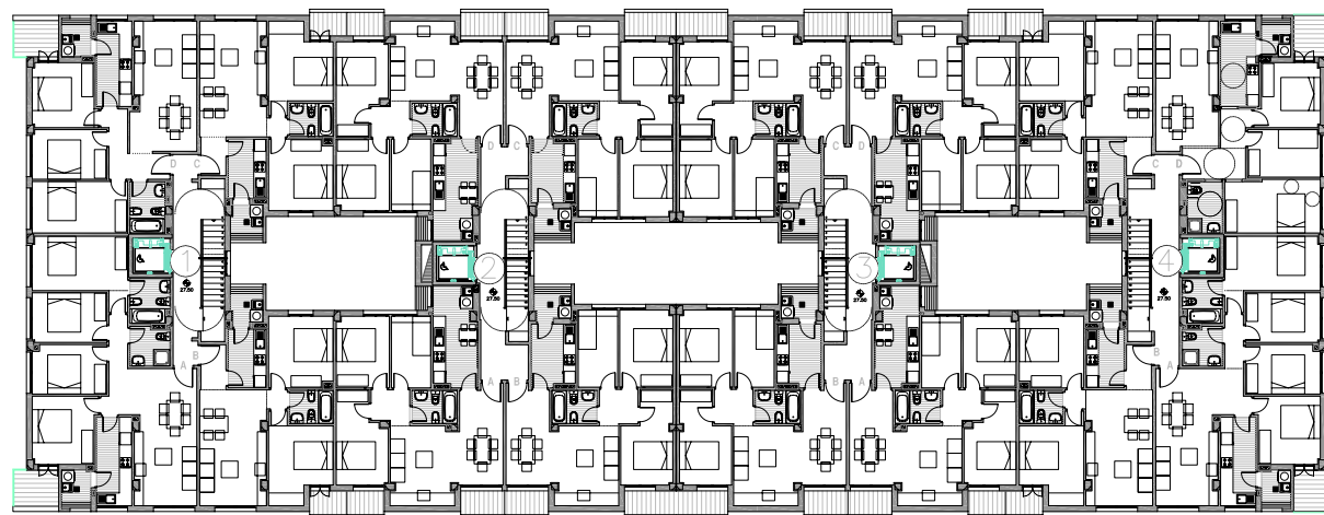
PLANTA TIPO
