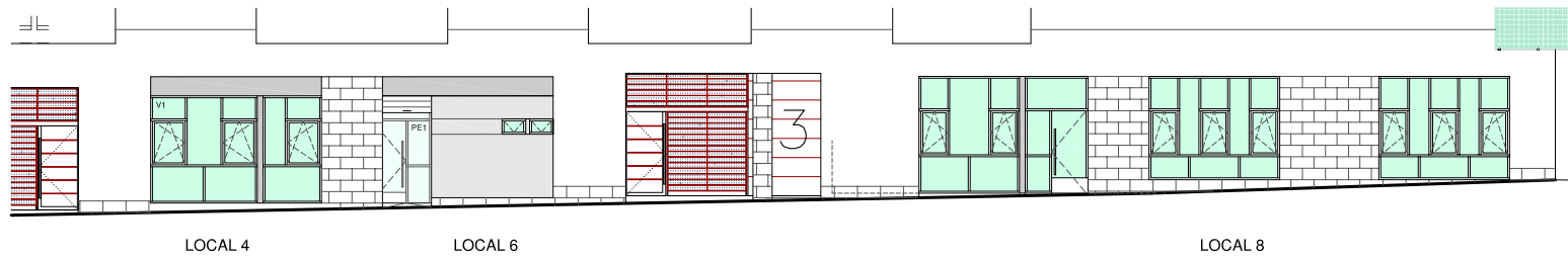
Alzado a Zona Verde
