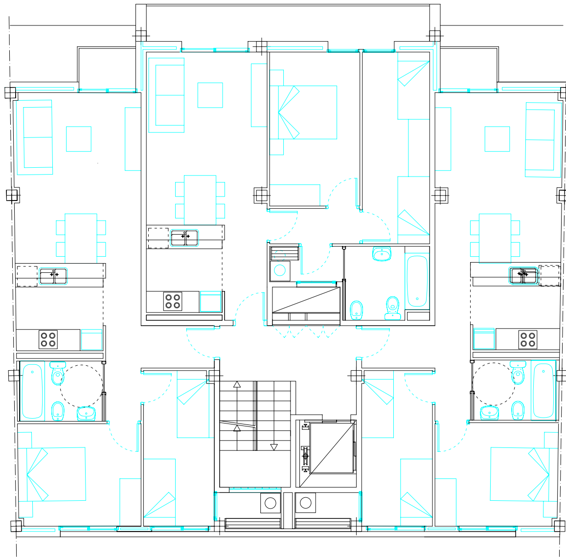
HABITATGES TIPUS AVDA. DELS PAISOS CATALANS
