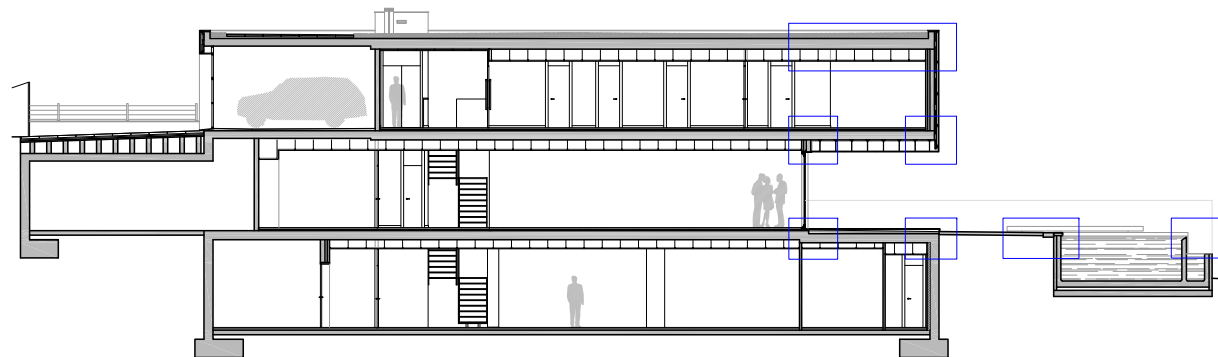
SECCIÓ LONGITUDINAL
