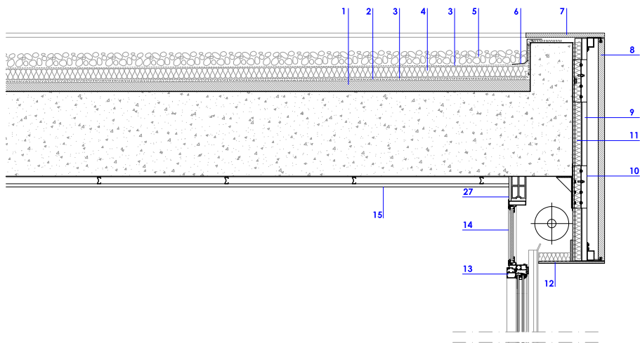
SECCIÓ LONGITUDINAL
