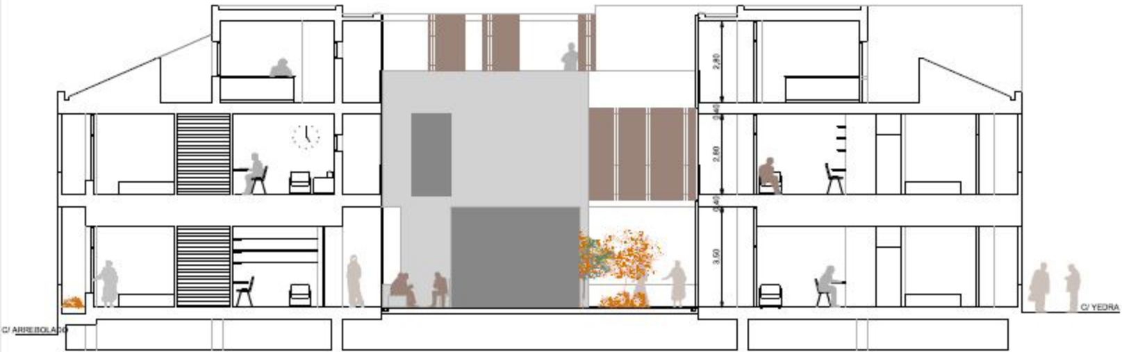
SECCIÓN C-D
