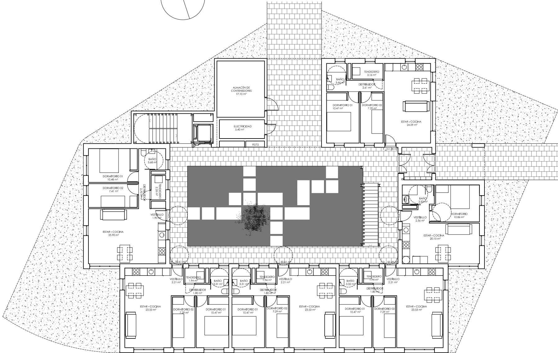
PLANTA BAJA
