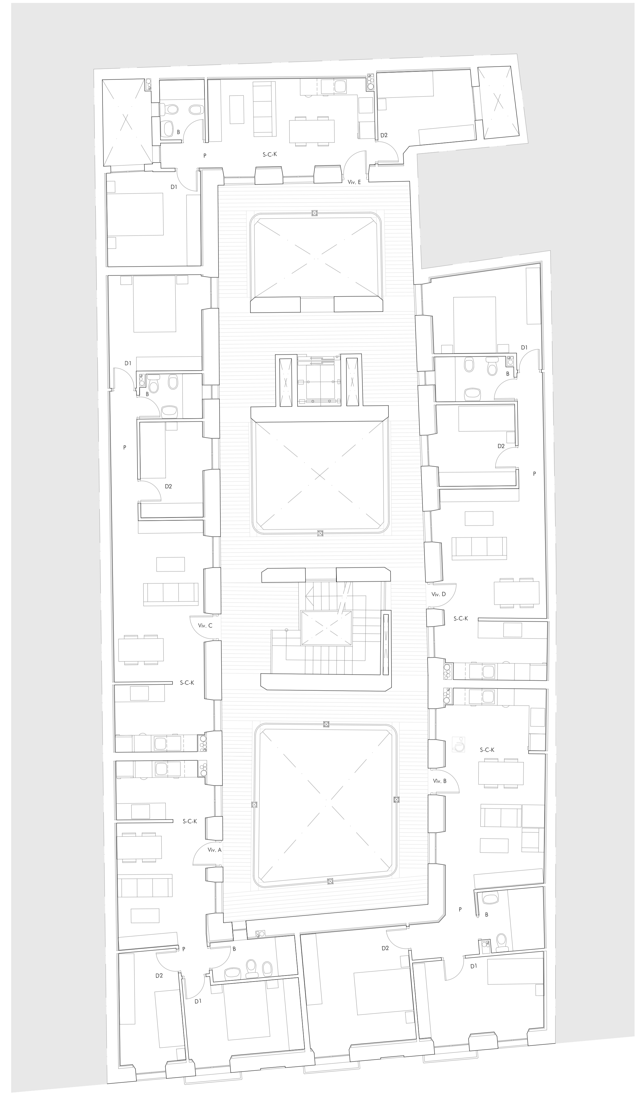
ESTADO REFORMADO PLANTAS PRIMERA Y SEGUNDA
