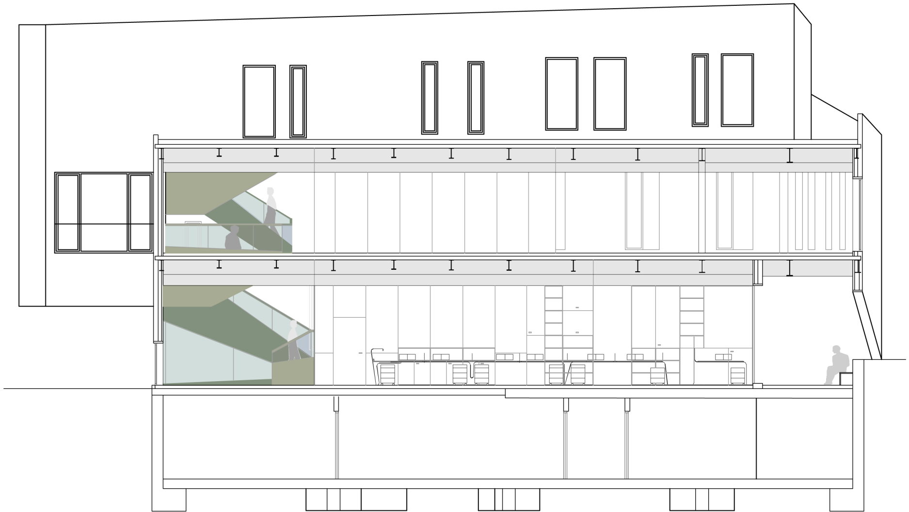
SECCIÓ LONGITUDINAL
