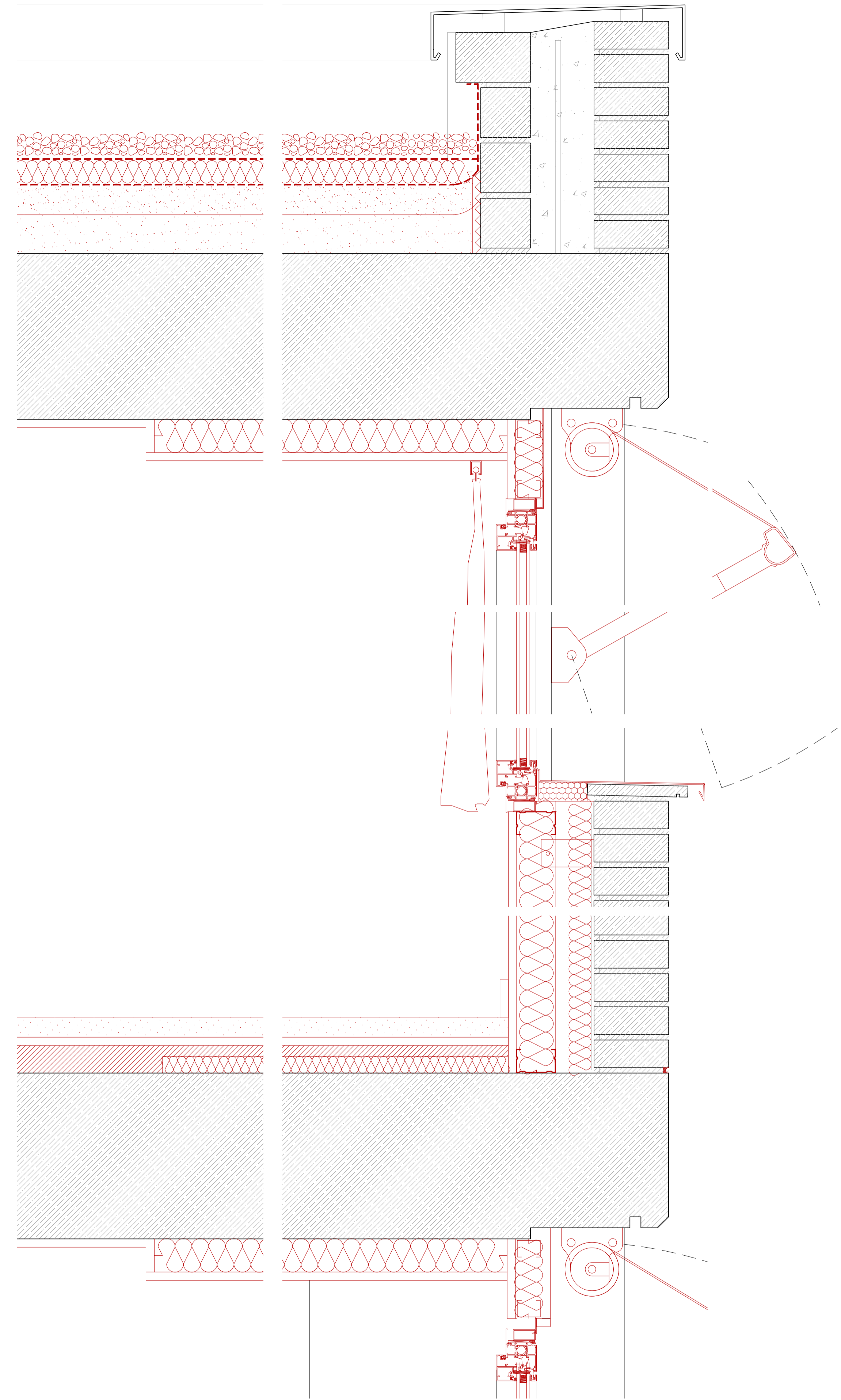
SECCIÓN CONSTRUCTIVA PROPUESTA
