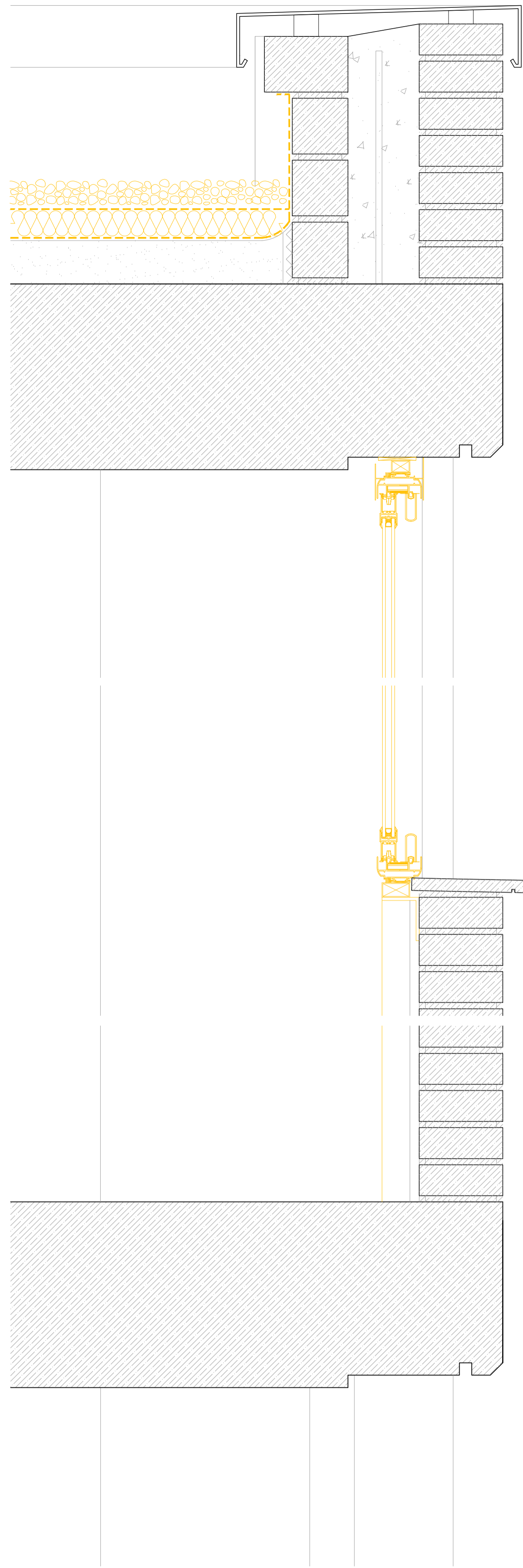
SECCIÓN CONSTRUCTIVA ESTADO PREVIO
