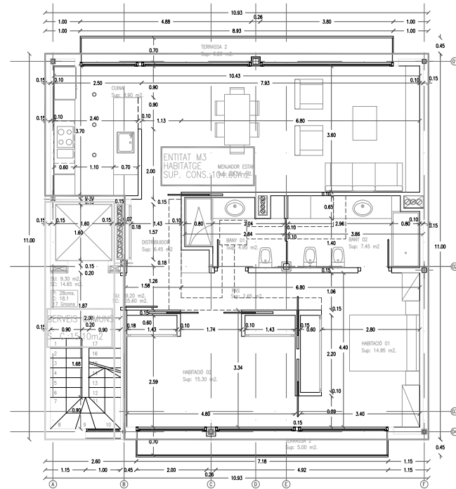
PLANTA SEGONA
