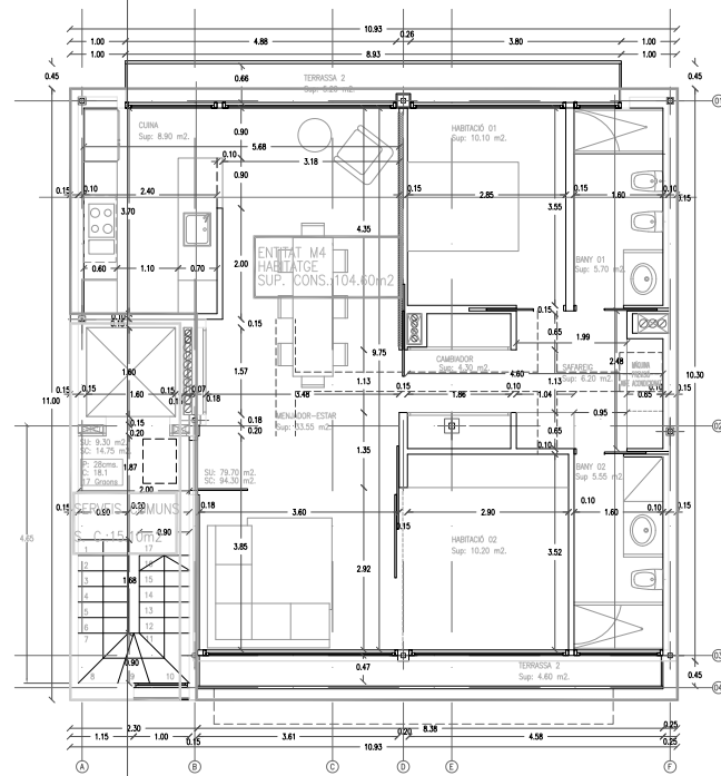
PLANTA TERCERA
