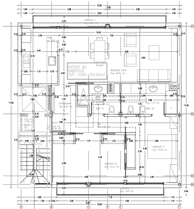
PLANTA PRIMERA
