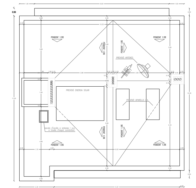
PLANTA COBERTA
