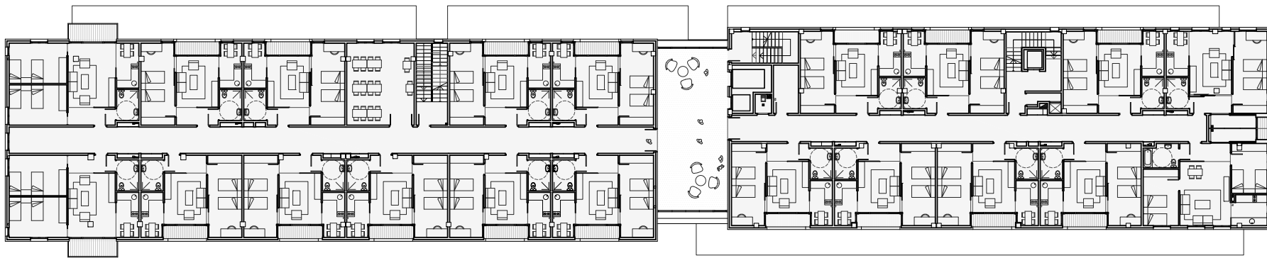
Planta TIPO (1ª, 2ª, 3ª Y 4ª) | Cota +4,20m (e: 1/500)
