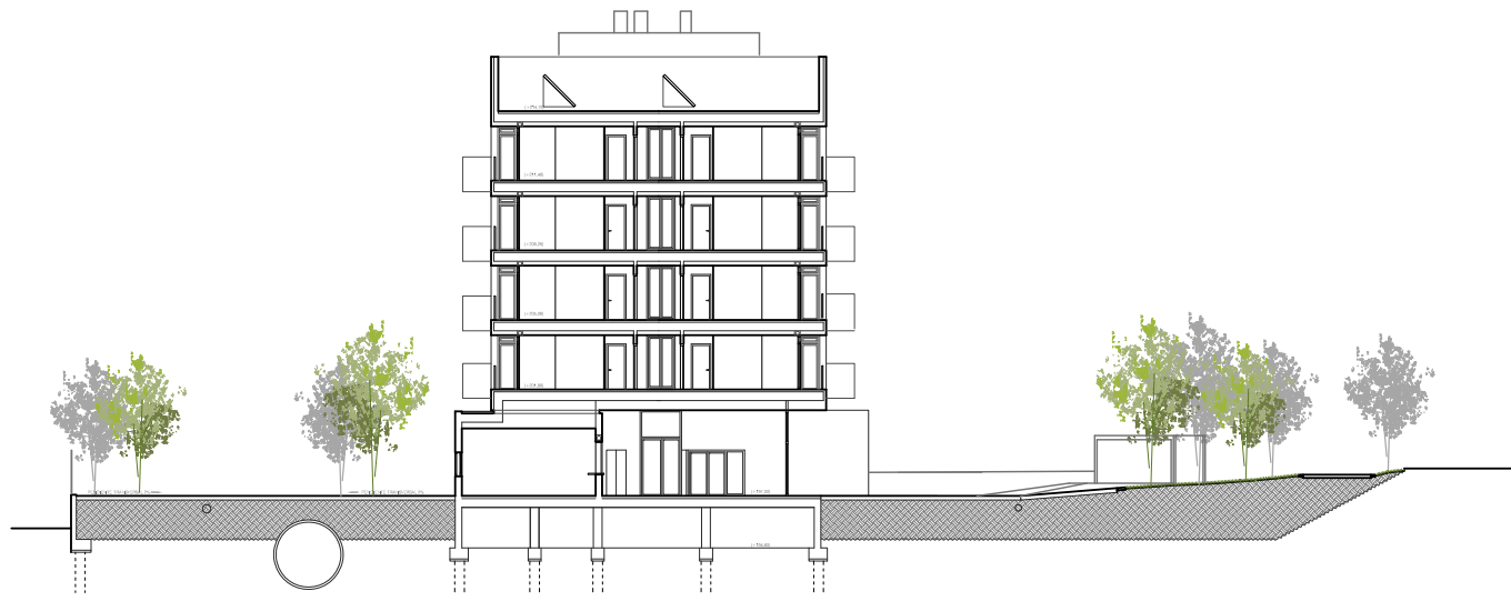
Sección TRANSVERSAL AA' | ACCESO + VIVIENDAS (e: 1/500)
