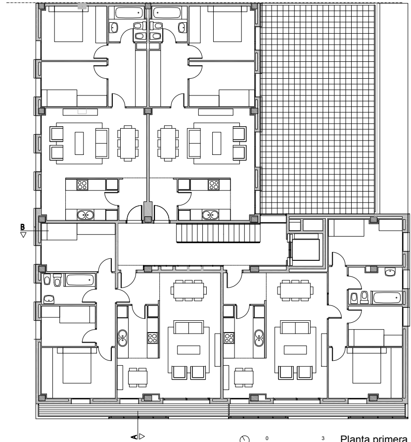
Planta primera
