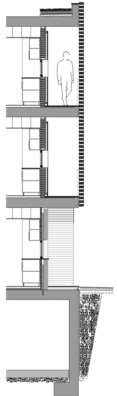
SECCIÓ CONSTRUCTIVA
