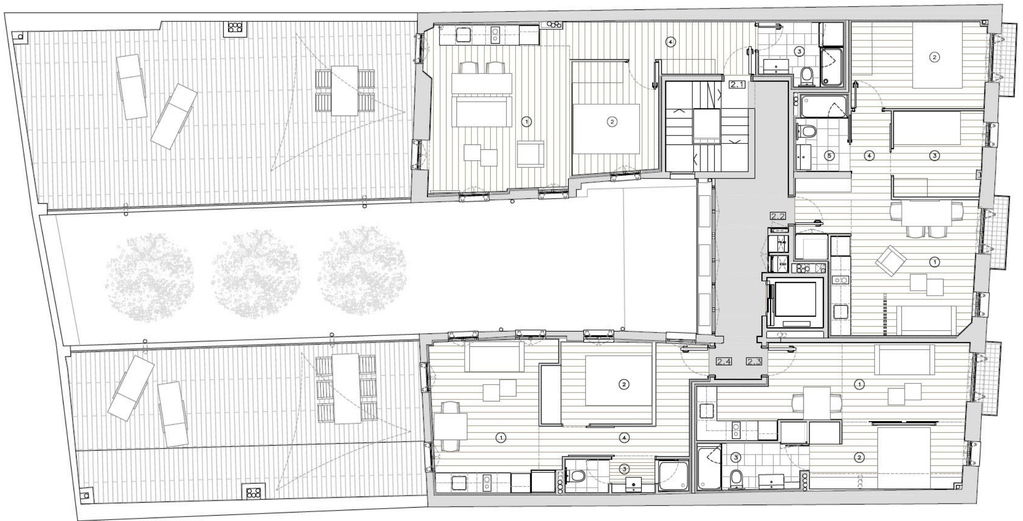
Planta 2
