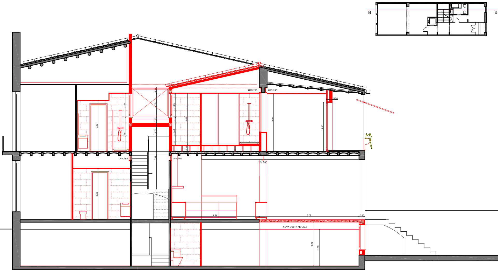
PARCEL·LA A SECCIÓ BB
