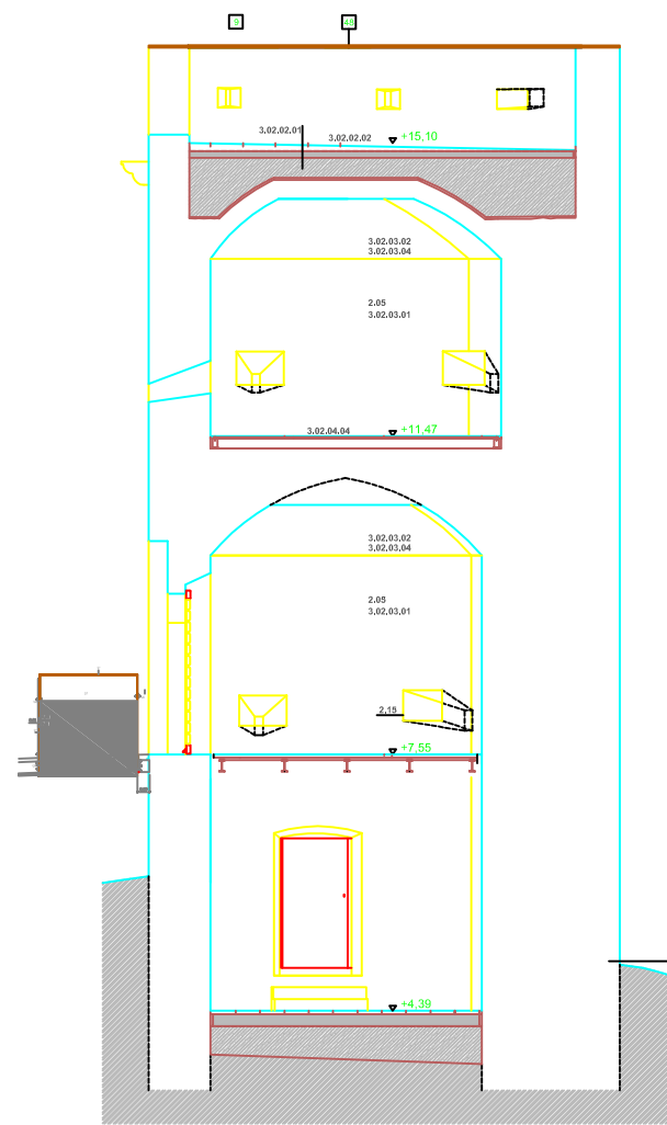
SECCIÓ LONGITUDINAL C-C'
