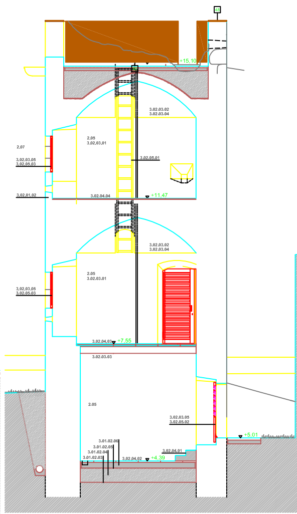
SECCIÓ TRANSVERSAL B-B'
