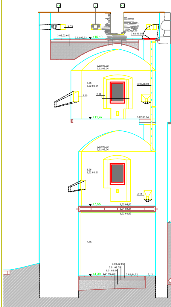
SECCIÓ LONGITUDINAL A-A'
