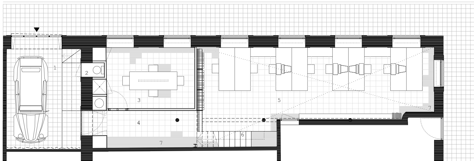
planta baixa
