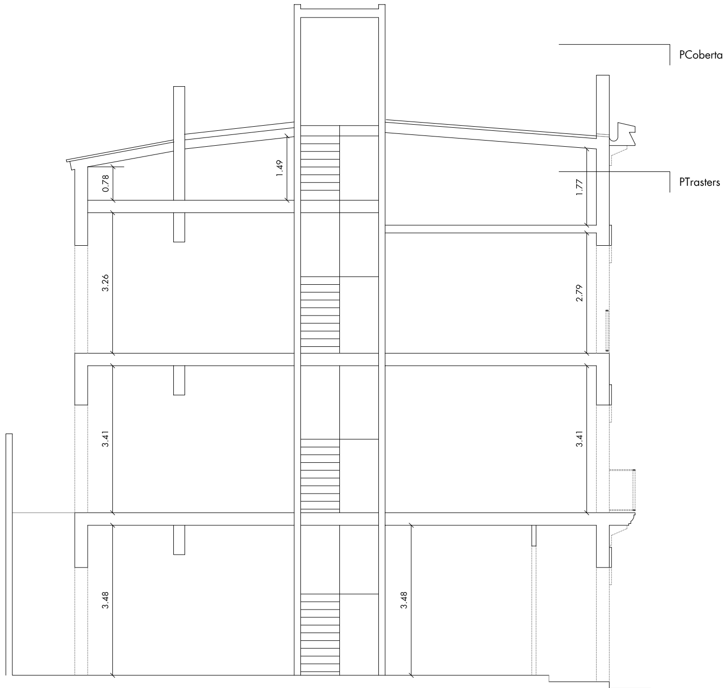
SECCIÓ LONGITUDINAL A
