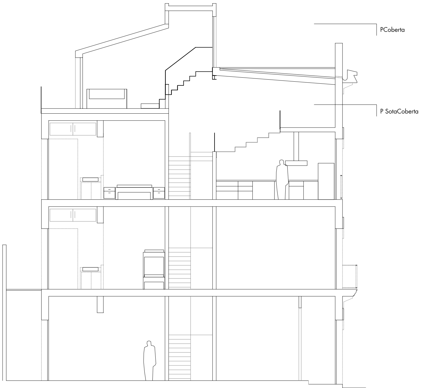
SECCIÓ LONGITUDINAL B
