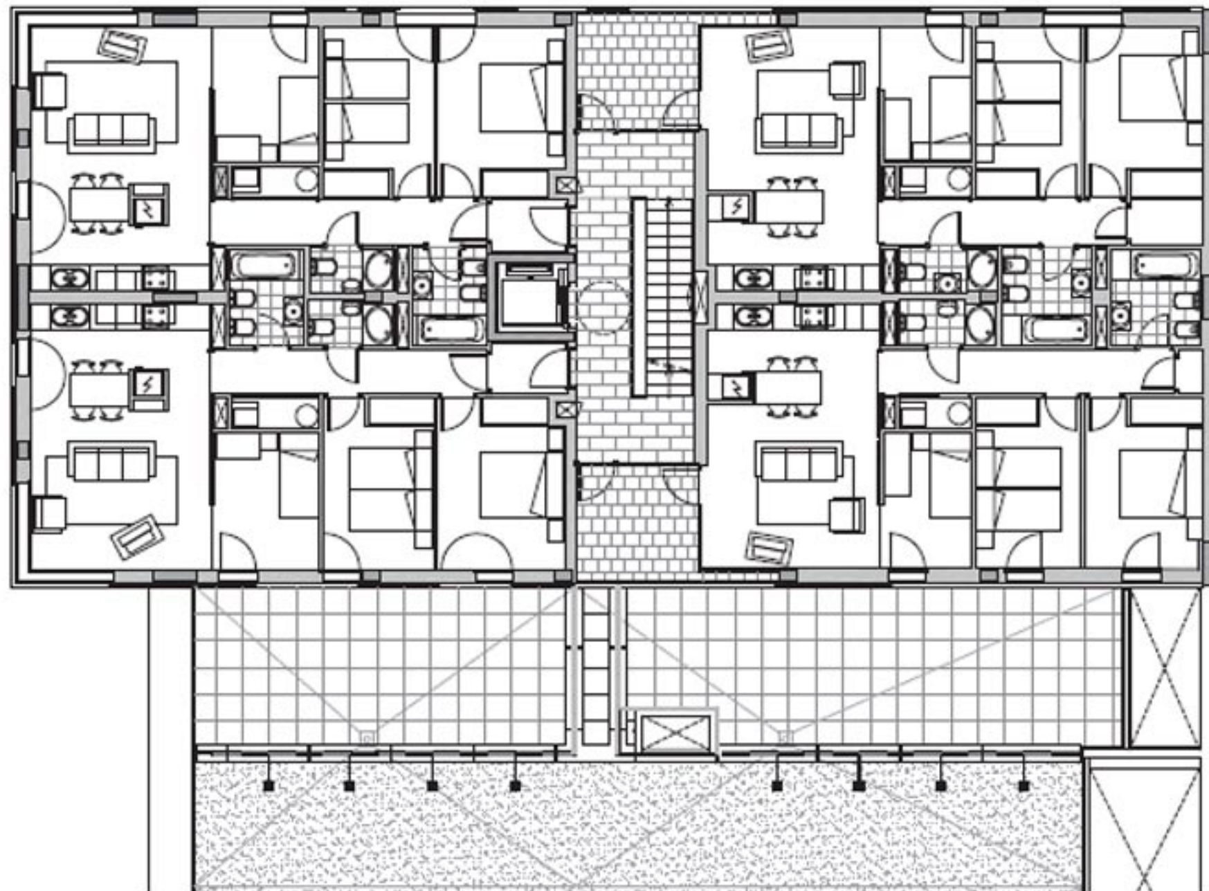
PLANTA TIPUS
