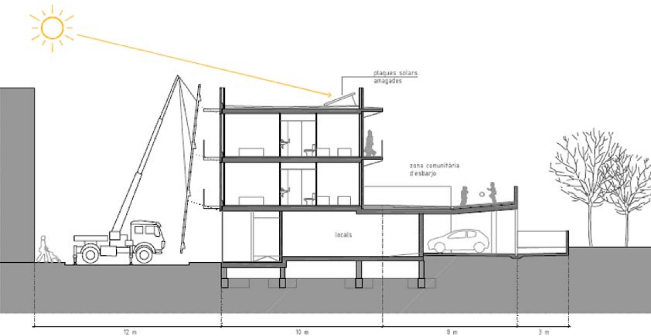
Secció transversal AA' 1/150
