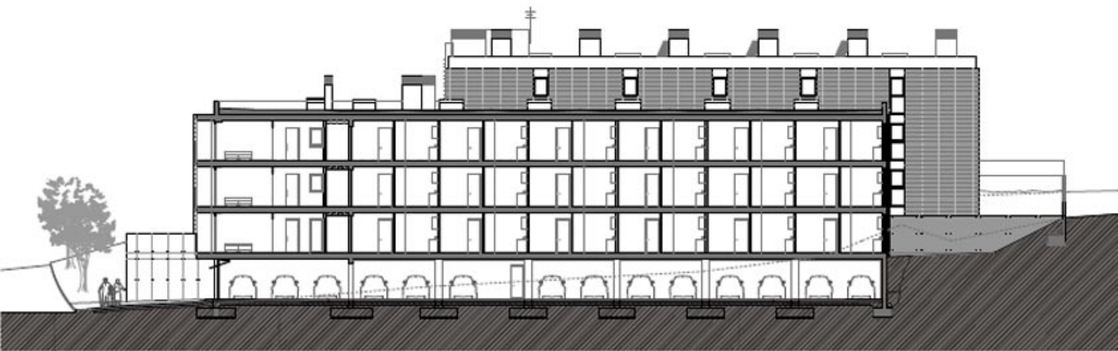
SECCIÓ LONGITUDINAL
