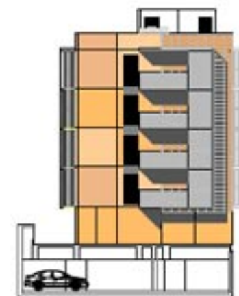
ALÇAT D-D' (1:200)
