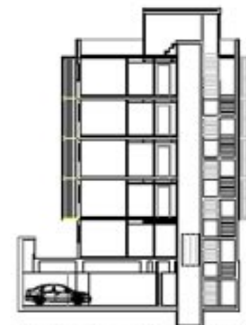
SECCIÓ D-D' (1:200)
