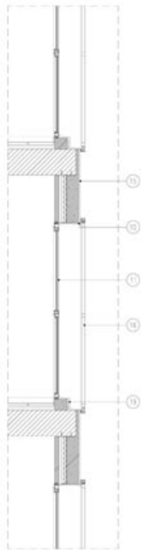
SECCÖ DETAY 1
