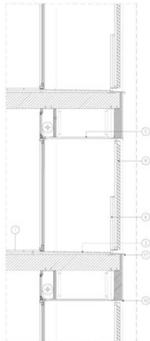
SECCÖ DETAY 2
