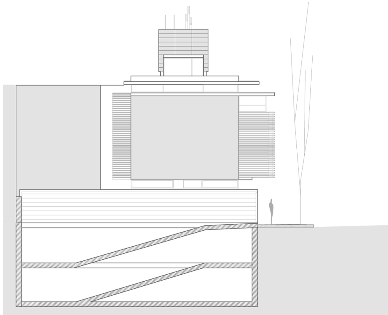
FAÇANA SUD
