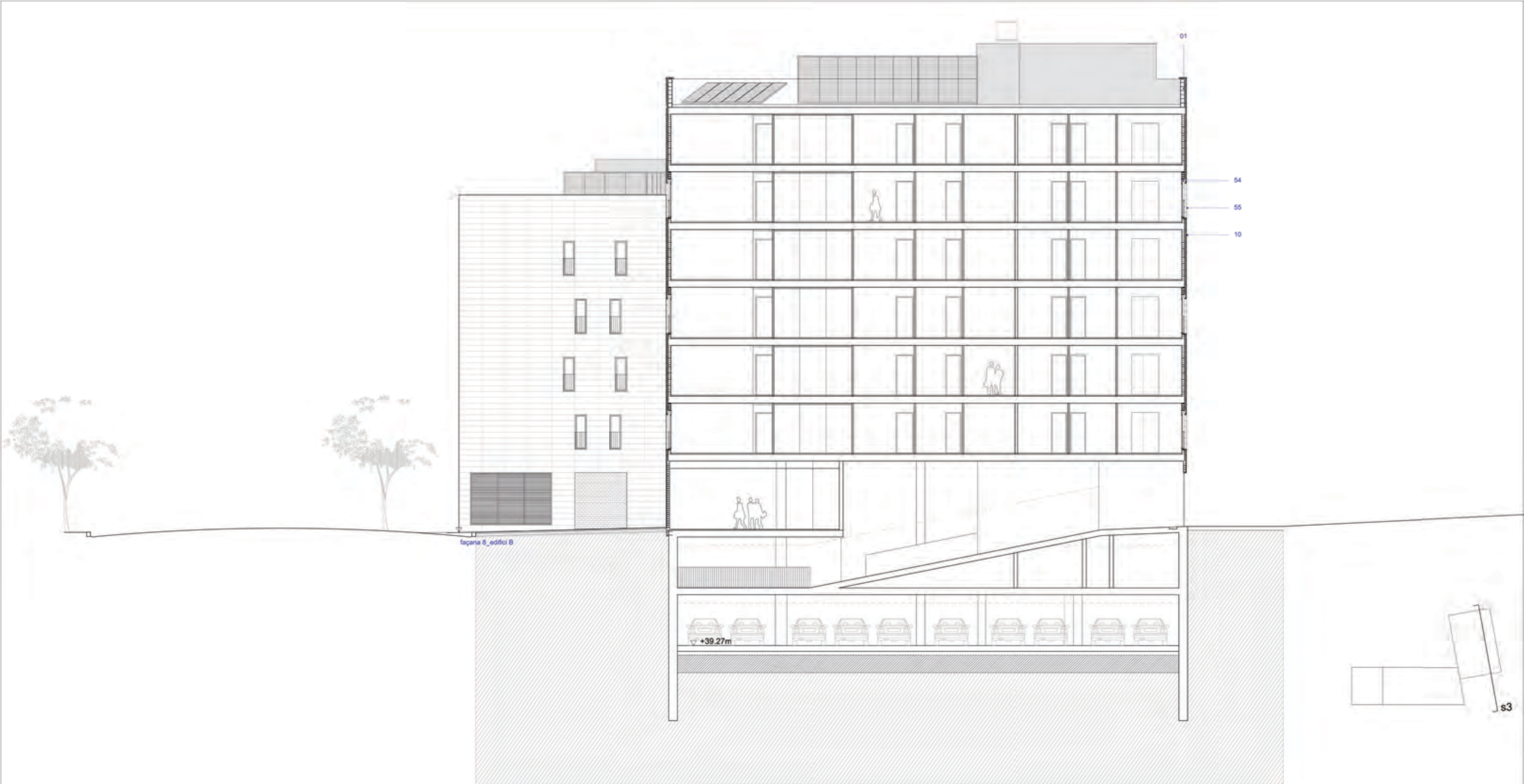
s3-secció longitudinal edifici A
