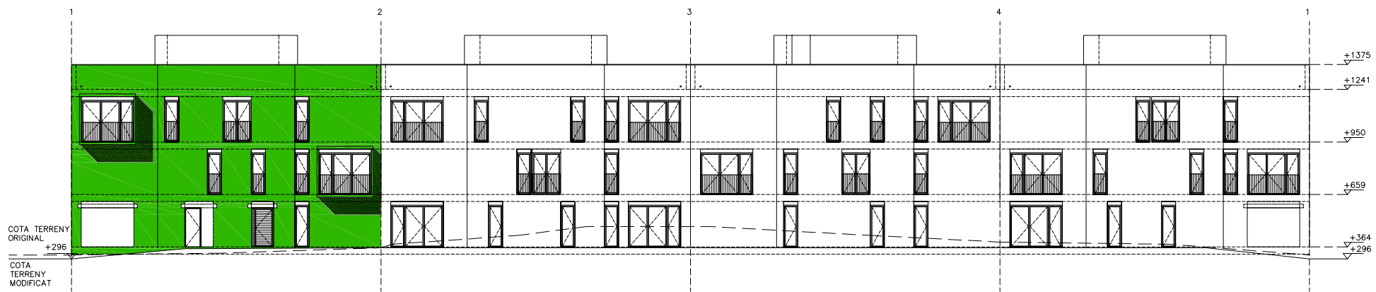
alzado bloque A - escala 1:150
