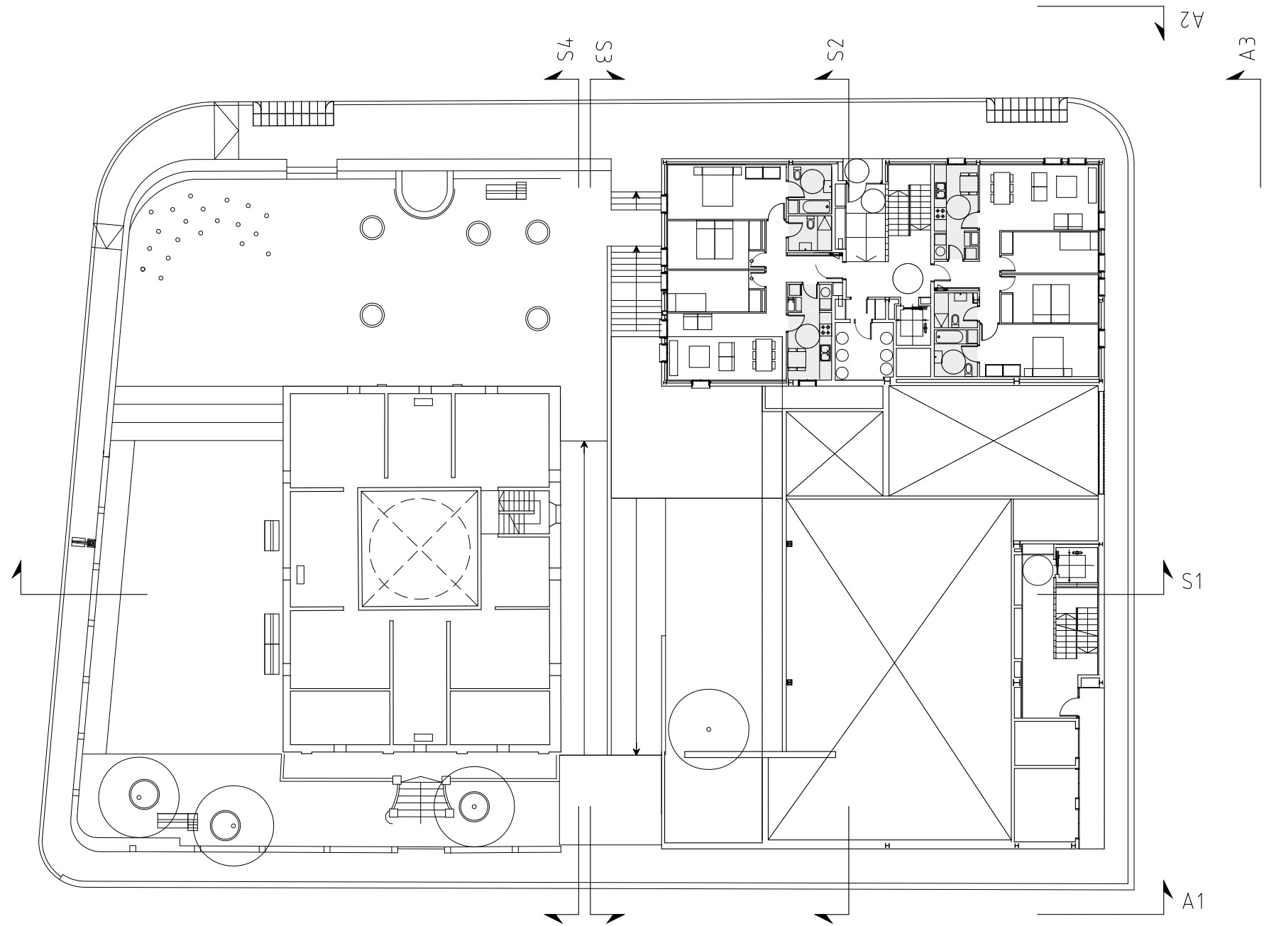
PLANTA BAIXA
