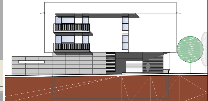
ALÇAT NORD. e.: 1/300
