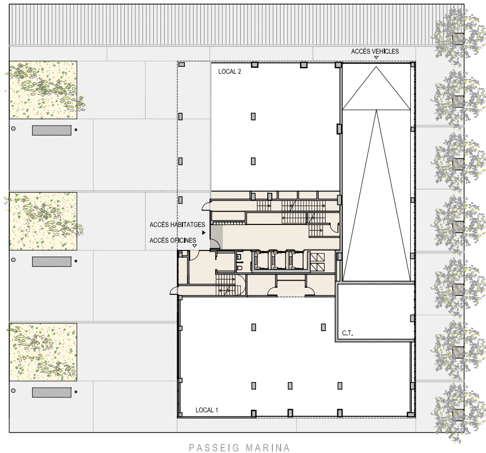
0 4 PLANTA BAIXA
