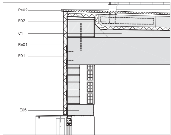
D.1 ENCUESTRO CUBIERTA/FACHADA
