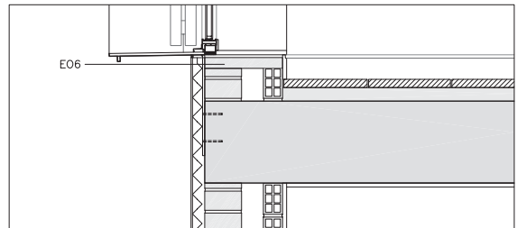
D.2 ENCUESTRO FORJADO/FACHADA
