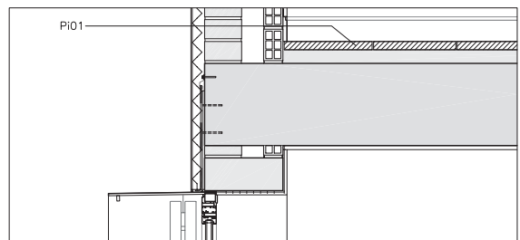
D.3 ENCUESTRO FORJADO/FACHADA
