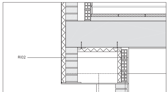
D.5 ENCUESTRO FACHADA/VOLADIZO
