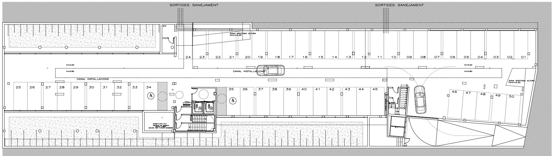
PLANTA SOTERRANI
