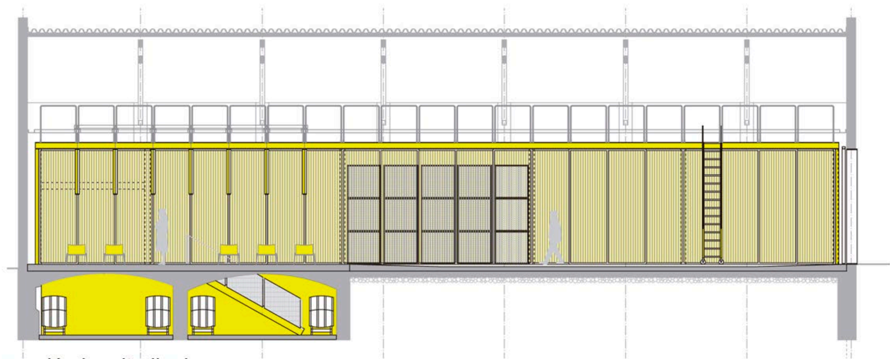
sección longitudinal
